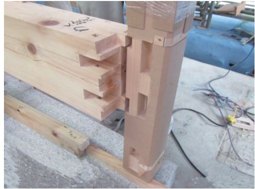
図17 茶室棟足固の仕口 隅
